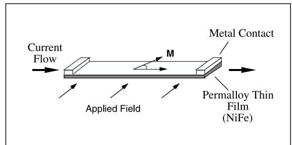
图1 磁阻传感器的工作原理
