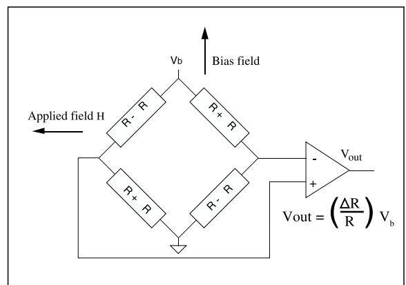
图2 磁阻传感器
