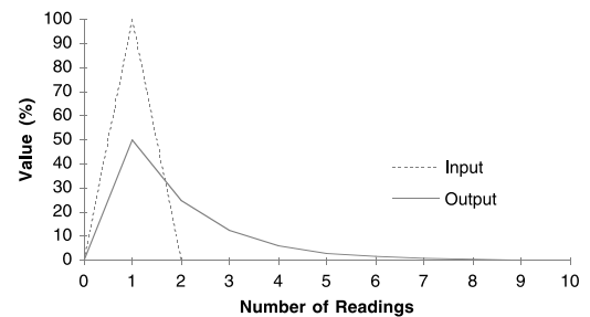
对于脉冲输入的平均读数响应
