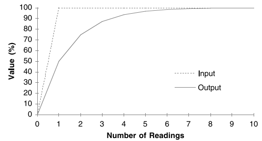
对于阶跃输入的平均读数响应
