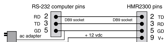
计算机RS-232和HMR2300的连接方法
