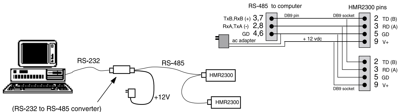
计算机 RS-485 和 HMR2300 的连接方法
