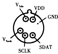
图 1 引脚说明
