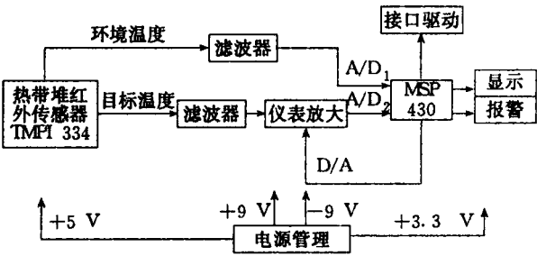
图 3 系统框图
