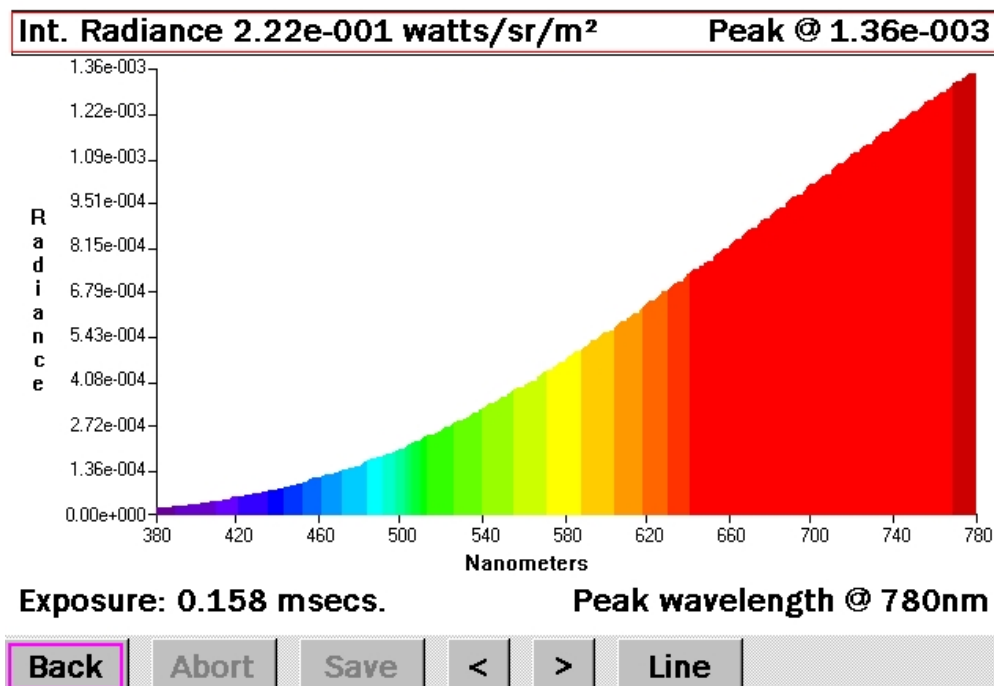
辐亮度图
