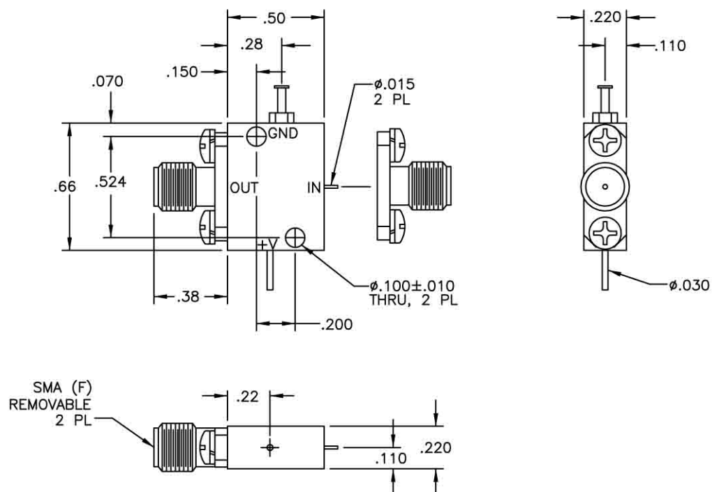
OUTLINE 0A
