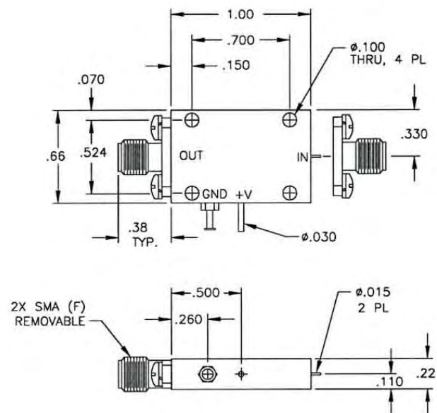
OUTLINE 2A
