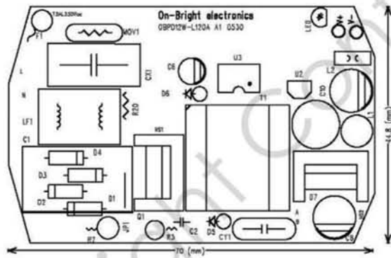
Top silk layer
