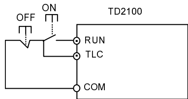
图6-22 三线运行控制模式
