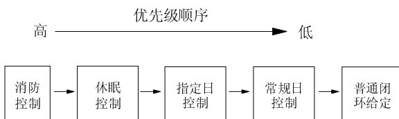
图7-3 控制功能优先级
