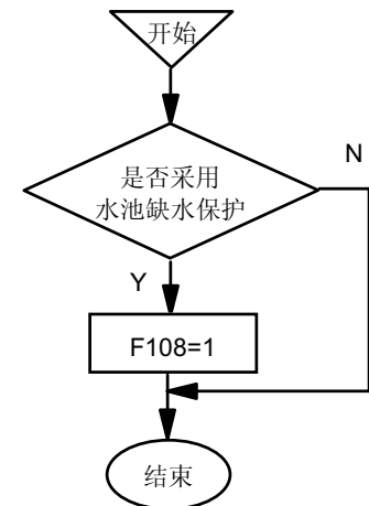
图7-10 缺水检测参数设置步骤
