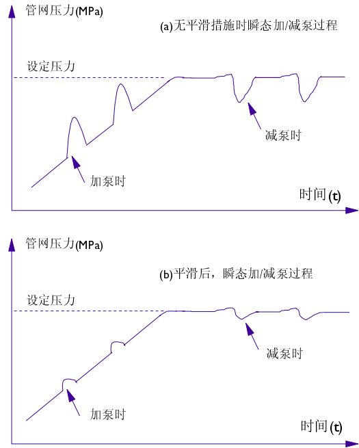
图6—12 有无平滑措施时加/减泵过程对比示意图
