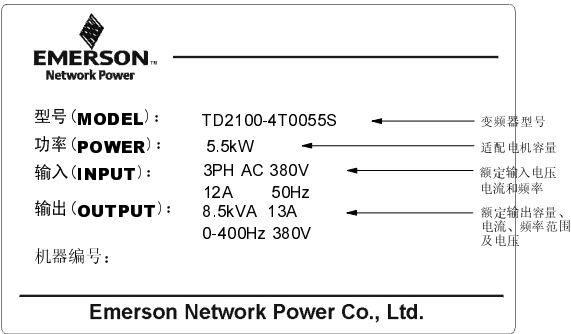
图1—1 变频器铭牌
