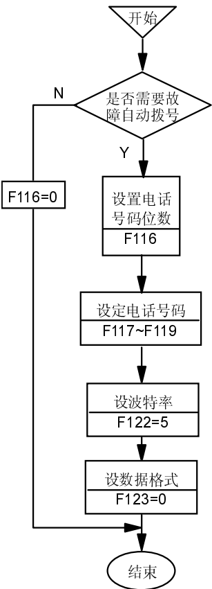
图7-11 故障自动拨号参数设置步骤
