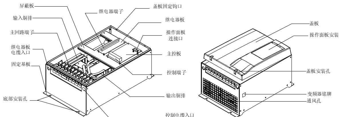
图1-3 变频器部件名称
