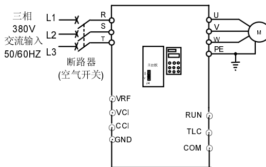
图3—6 基本配线图
