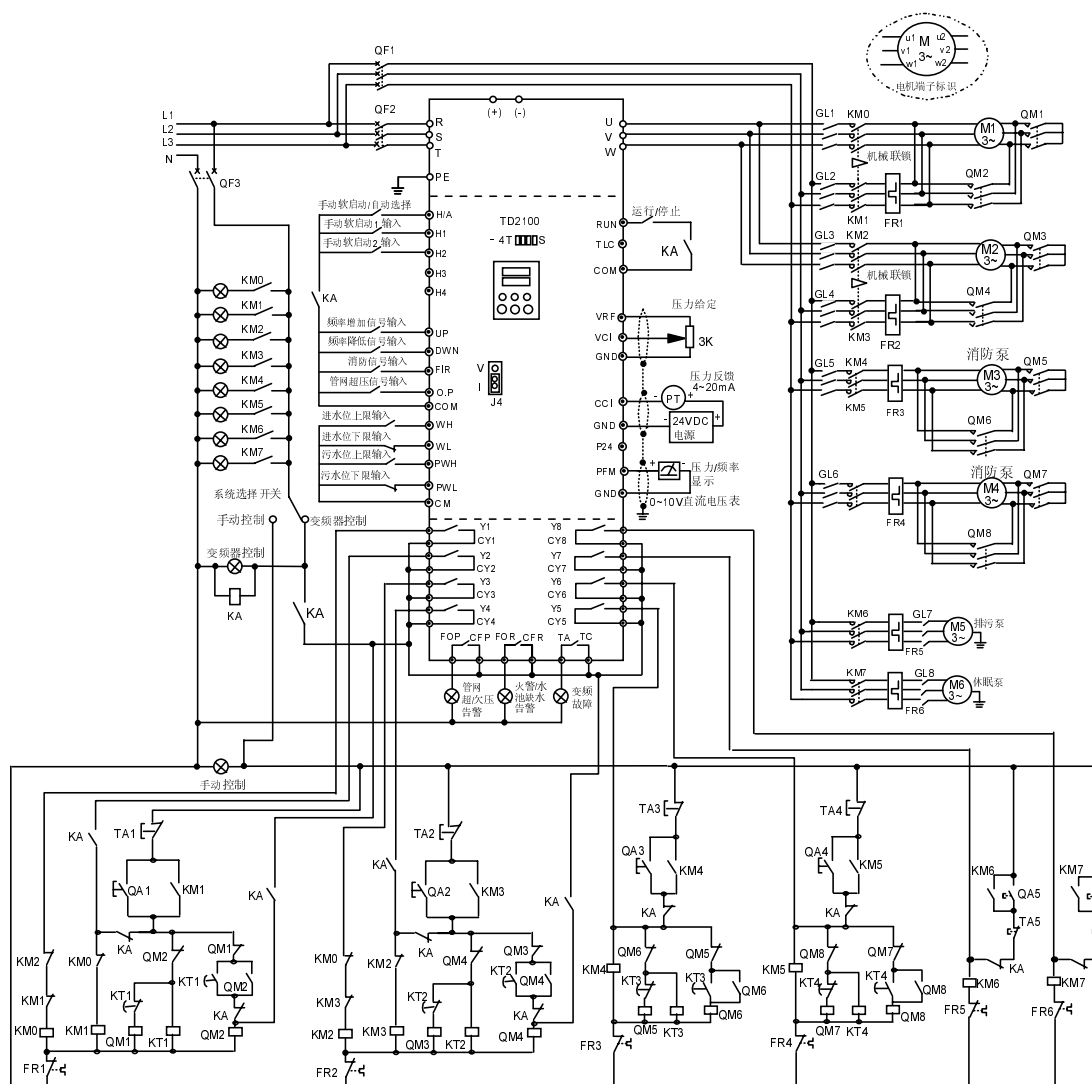
图3-17 带2台常规泵的变频循环方式（2个常规泵一用一备方式，具备Y- \Delta 启动控制功能）
