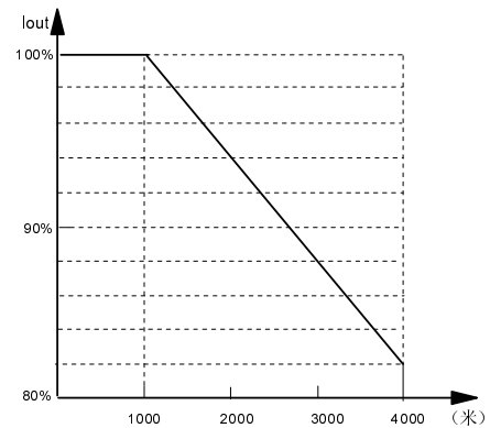
图1-6 变频器额定输出电流与海拔高度降额关系
