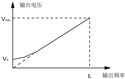
图6-3 手动转矩提升
