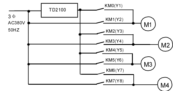
图6-11 F25=3或7（4泵变频循环方式）最大配置示意图
