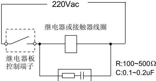
图3—7a RC 阻容吸收电路
