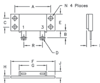
TO-249 Non Isolated
