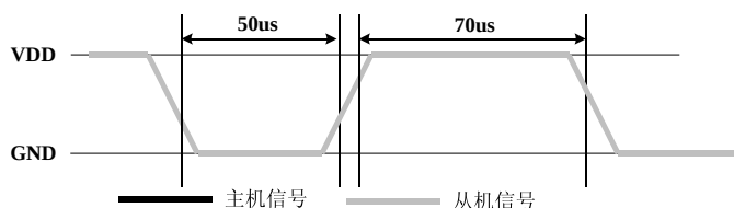
位数据“1”格式
