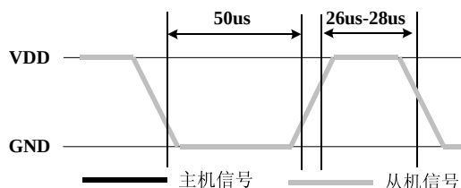
位数据“0”格式
