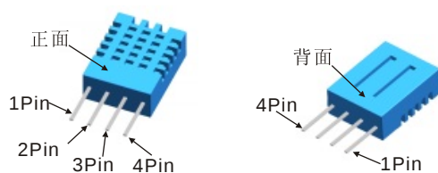
AM2302引脚图
