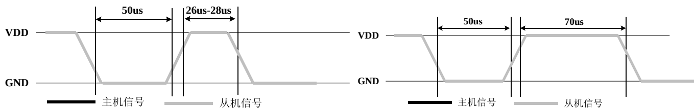
位数据“0”格式
