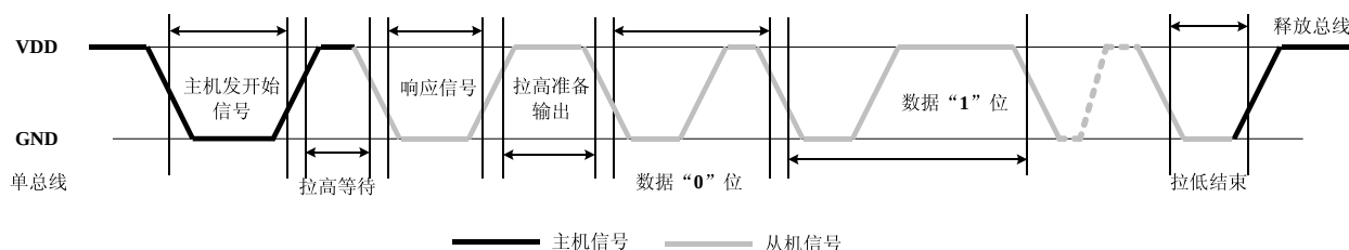
数据时序图
