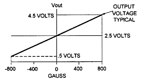
输出曲线 @ V_s=5.0VDC
